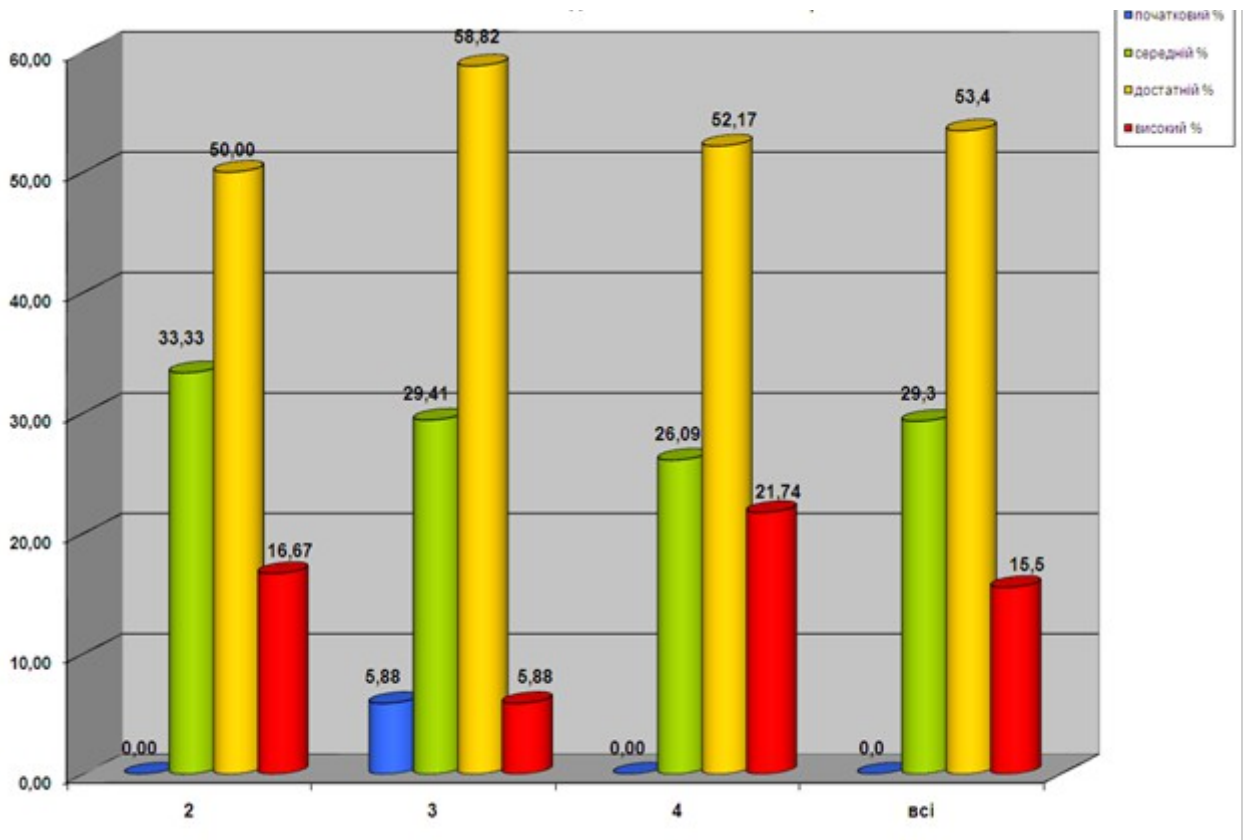
Малюнок 1: Рівні навчальних досягнень за 2013-2014 н.р.
